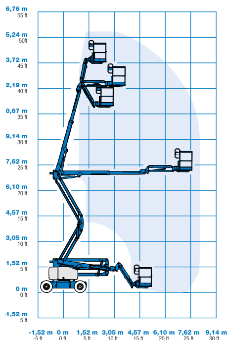
Diagrama de trabajo Z-45/25J
