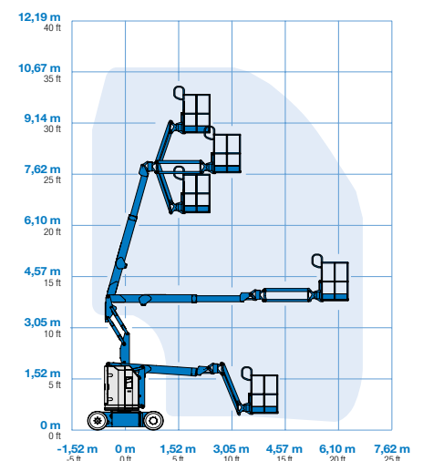
Diagrama de trabajo del plumín Z-30/20N RJ
