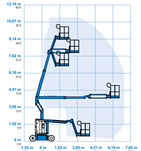
Diagrama de trabajo Z-30/20N
