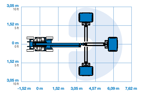
Diagrama de trabajo del plumín Z-30/20N RJ
